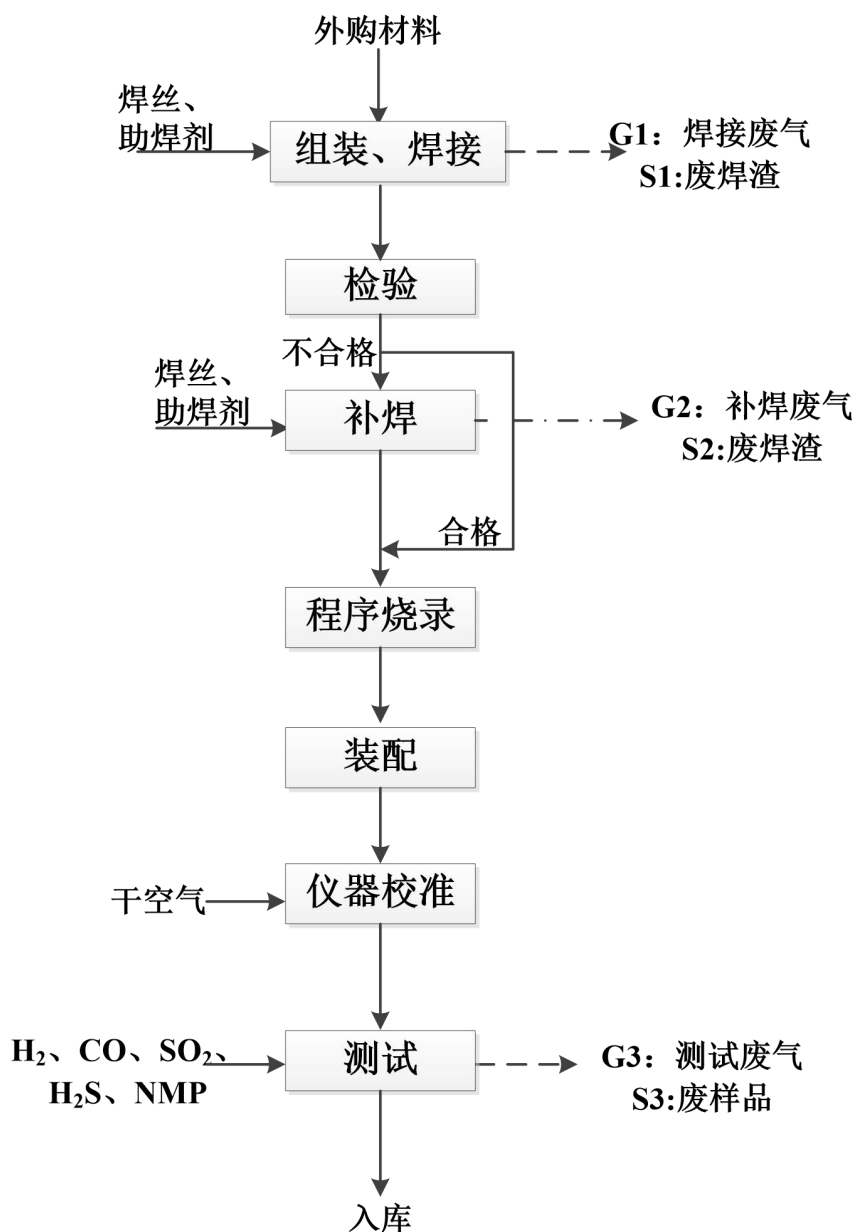
图 2-2 气体浓度检测仪研发及产污环节图
